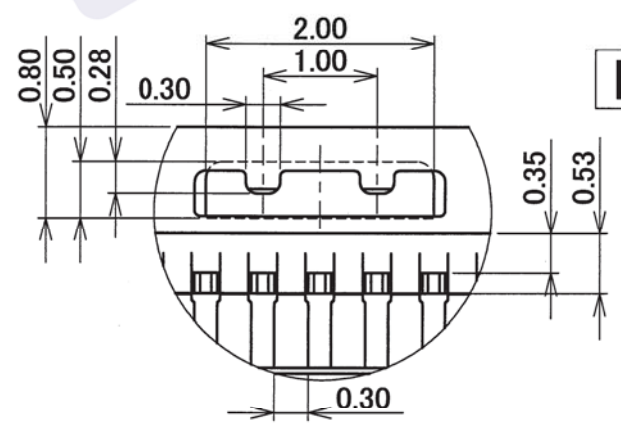
DETAIL L S= 15 : 1
